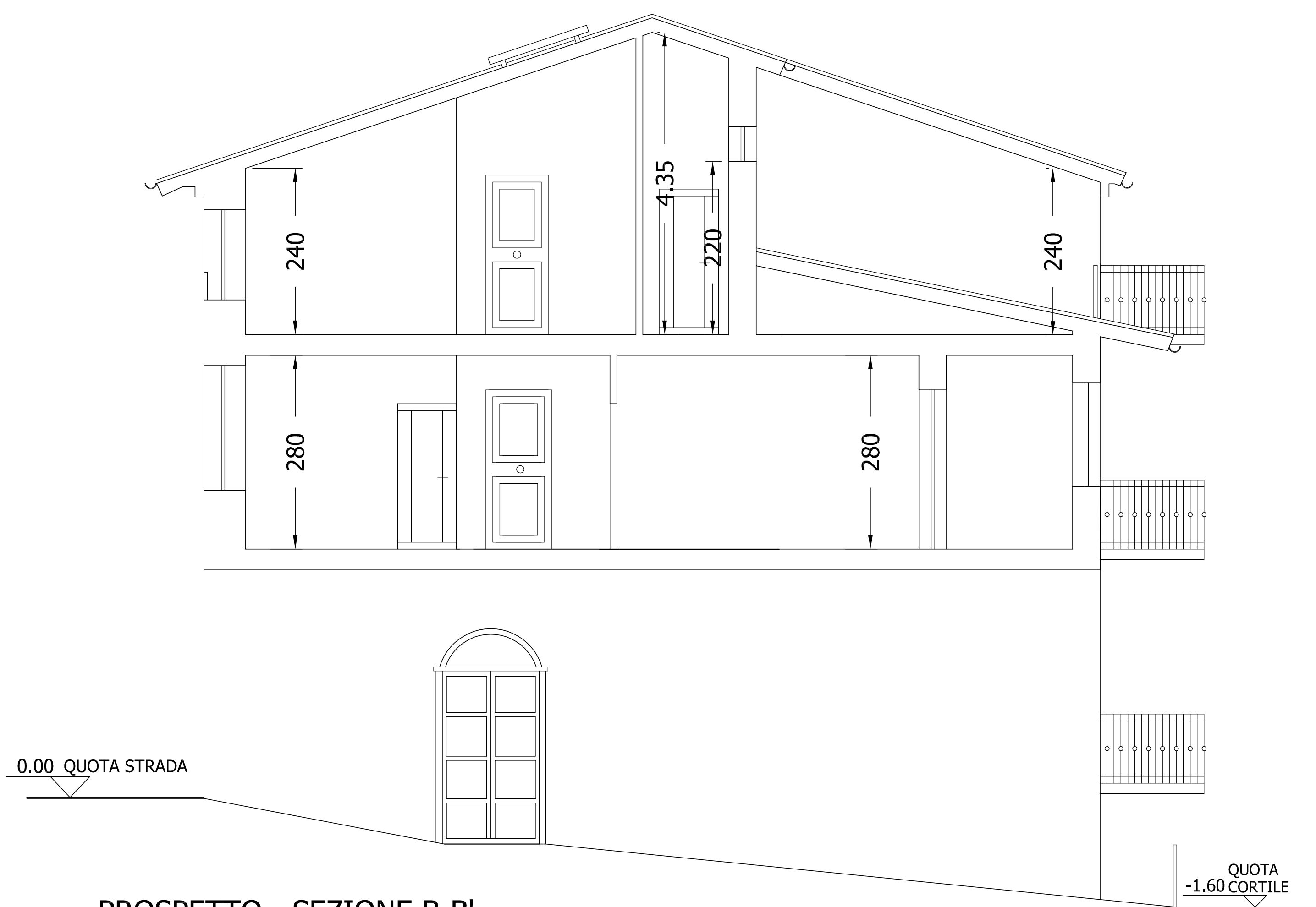
PROSPETTO - SEZIONE B-B'
