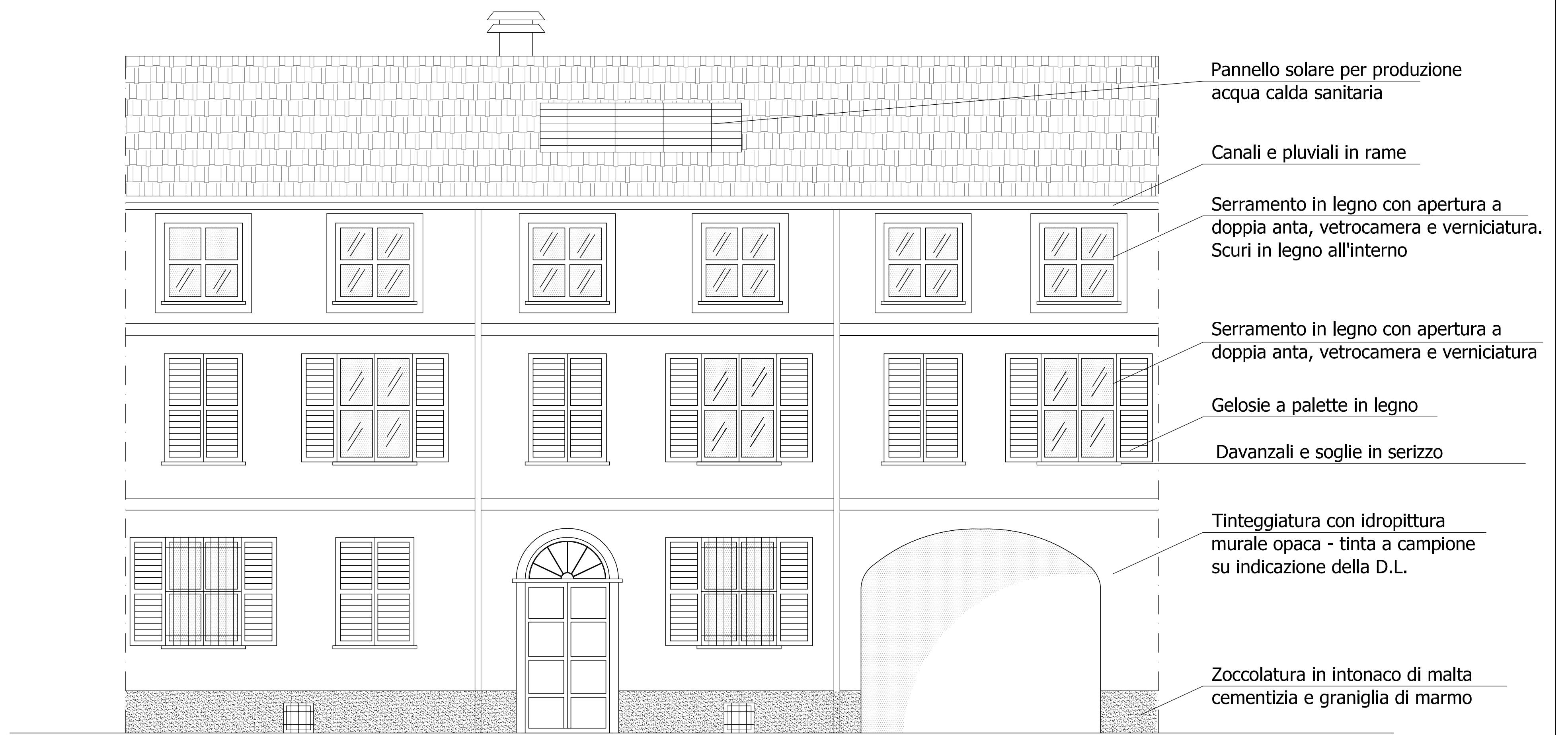
PROSPETTO SU VIA UMBERTO I°
